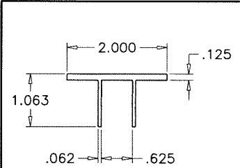
1R RAILING TOP COVER
